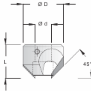
Зенкера
