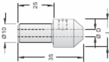
Быстросменные патроны
