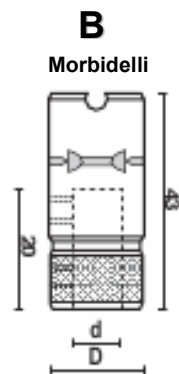
Быстросменные патроны
