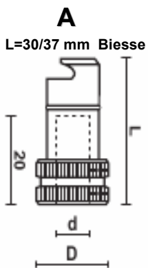
Быстросменные патроны
