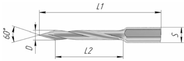
Твердосплавные сверла для сквозных отверстий
